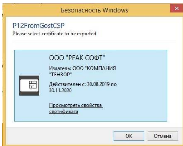
Рисунок 169 – Выбор сертификата
