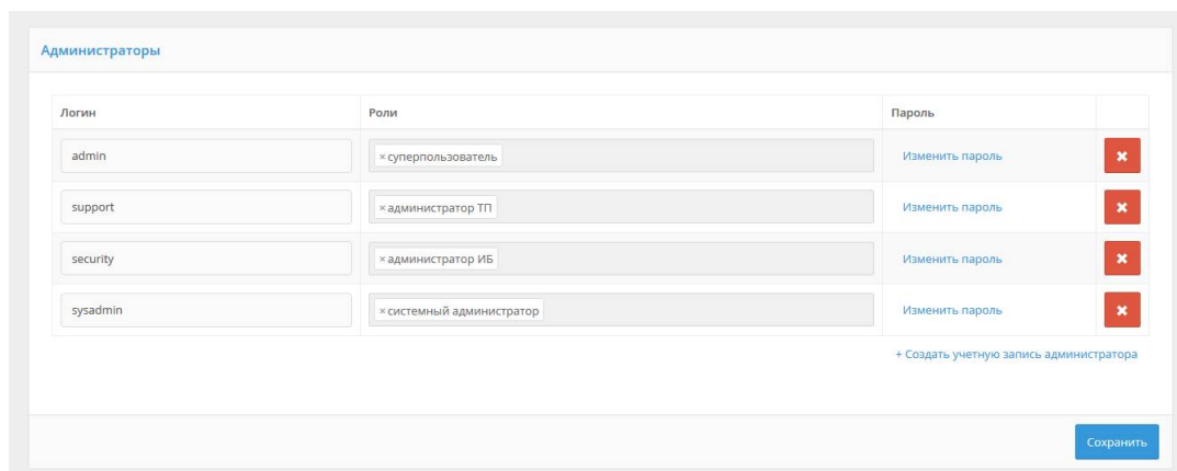
Рисунок 6 – Управление администраторами
