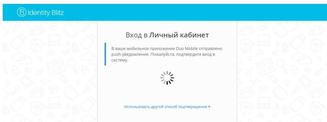
Рисунок 51 – Инициирование push-аутентификации
