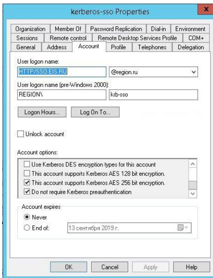
Рисунок 31 – Свойства Kerberos
