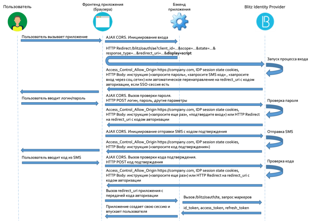
Рисунок 10 — Схема взаимодействия при входе по логину и паролю
