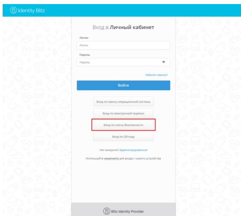
Рисунок 20 – Вход с использованием ключей безопасности
