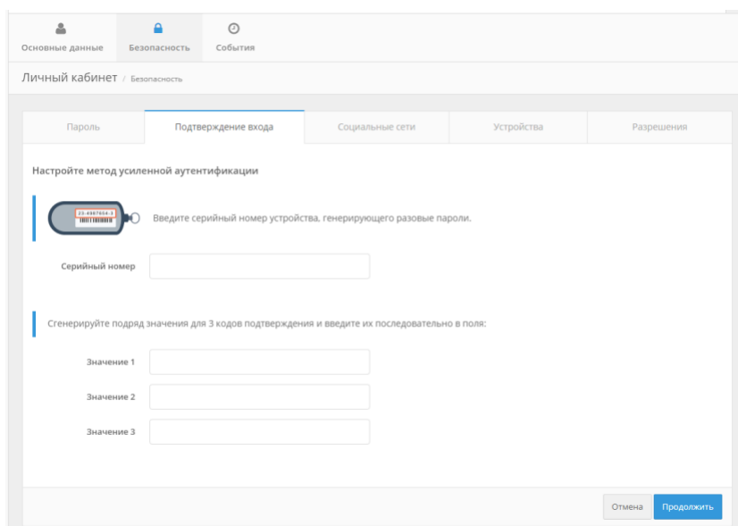
Рисунок 34 – Привязка специального устройства для генерирования разовых кодов
