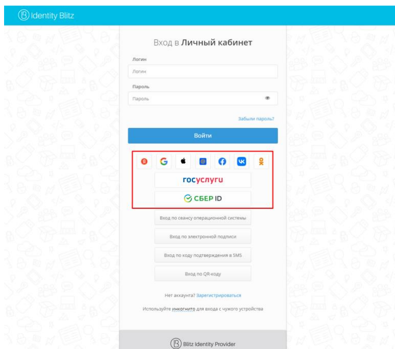
Рисунок 15 – Вид экрана входа при включенных внешних сервисах идентификации
